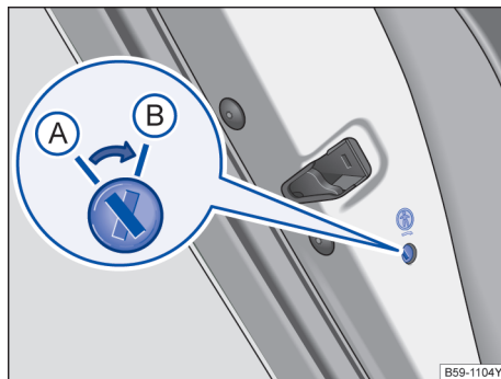
图 55 在左后车门中：儿童安全锁 A 已关闭、B 已接通
