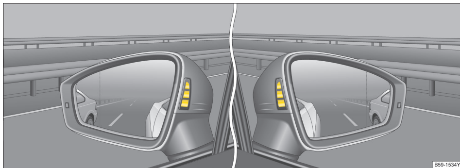
图 129 车外后视镜壳体上：变道辅助指示灯显示
