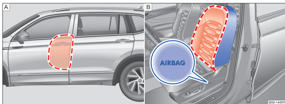
图 40 [A] 汽车左侧 - 侧面安全气囊膨胀范围 [B] 左前座椅侧面 - 侧面安全气囊安装位置及膨胀范围
