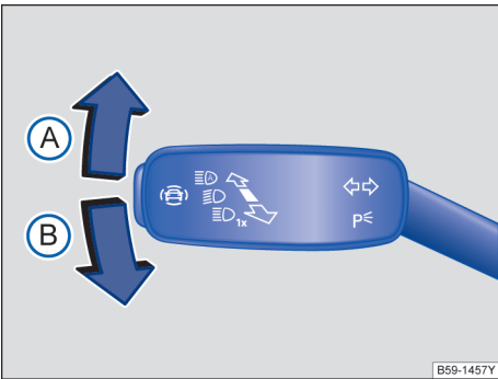
图 86 变道转向灯 / 远光灯操作杆
