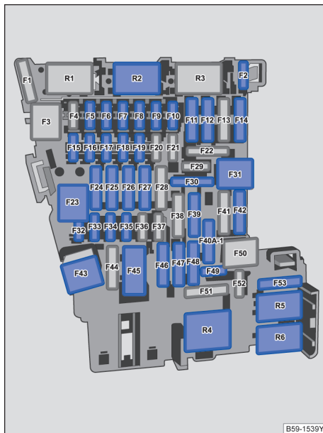
图 201 仪表板中：保险丝位置示意图
