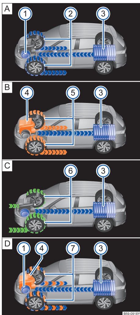
图 23 混合动力车型信息娱乐系统:能量流显示
