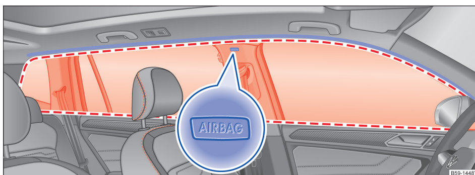
图 41 在汽车左侧：头部安全气囊的安装位置和膨胀范围
