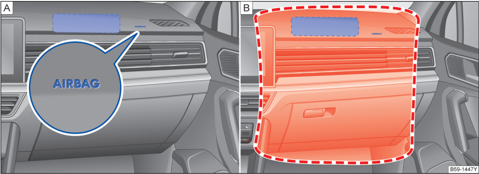
图 39 副驾驶员前部安全气囊的安装位置和膨胀范围
