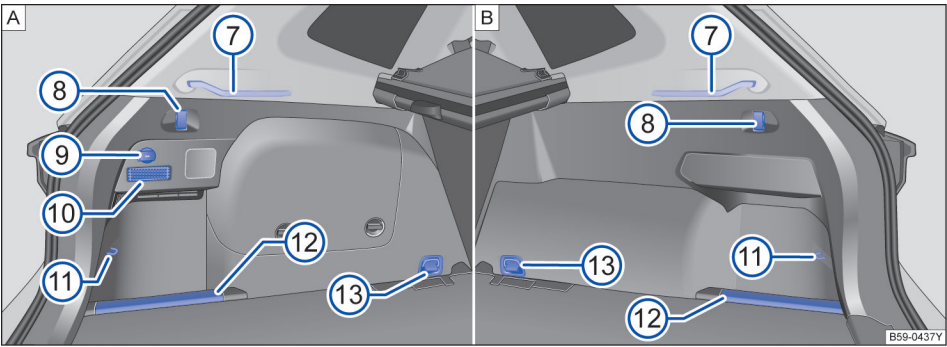
图 8 行李厢侧面区域
