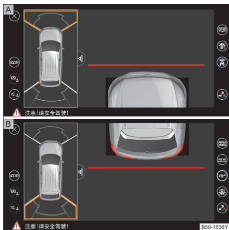
图 149 车周视野显示: A 前部摄像头, B 后部摄像头
