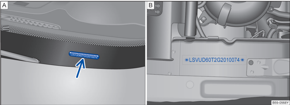
图 230 [A]. 车辆识别代号 [B]. 发动机舱内的车辆识别代号钢印位置
