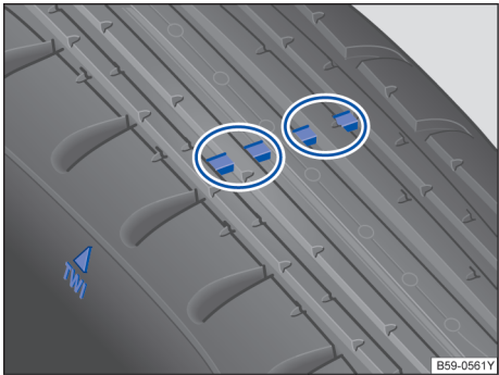
图 220 轮胎花纹磨损标记
