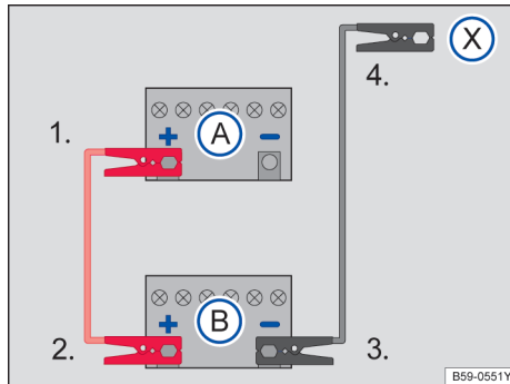
图 206 跨接电缆连接示意图
