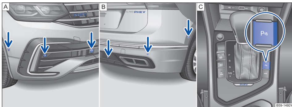
图 140 A 、 B 前后泊车雷达系统超声波传感器 C 开启或关闭泊车雷达系统的按钮（依装备而定）
