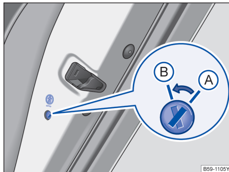
图 56 在右后车门中：儿童安全锁 A 已关闭、B 已接通
