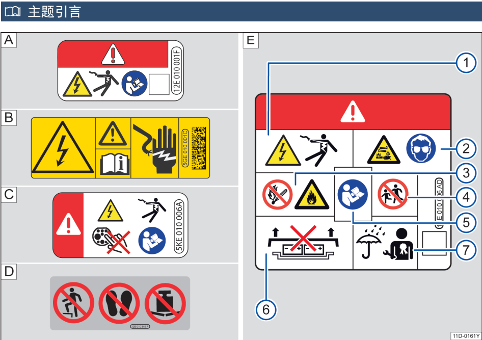
图 185 警告牌（示意图）：[A]. 高压组件 [B]. 高电压普通警告牌 [C]. 充电口高压警示标签 [D]、[E]. 高压电池上的警告牌
